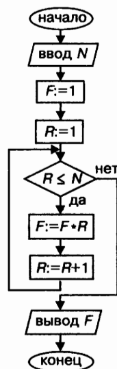
Рис. 6.7. Блок-схема алгоритма вычисления факториала
