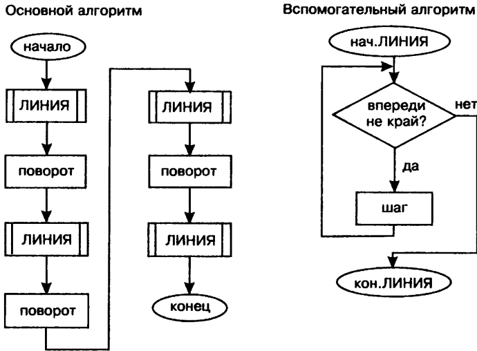
Рис. 5.8. Блок-схема алгоритма «Рамка»
