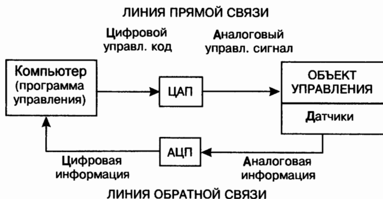
Рис. 5.16. Схема системы автоматического управления
