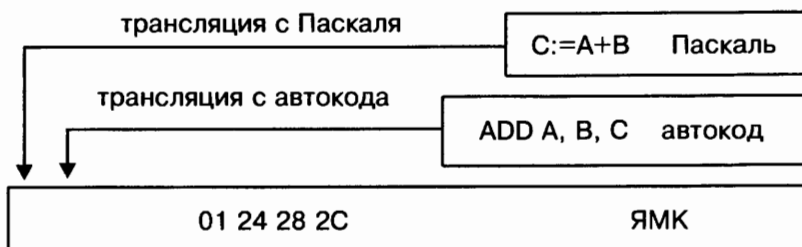
Рис. 6.18. Трансляция с автокода и Паскаля на ЯМК
