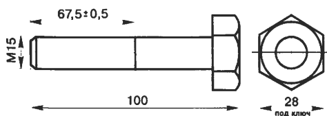
Рис. 2.3. Чертеж болта
