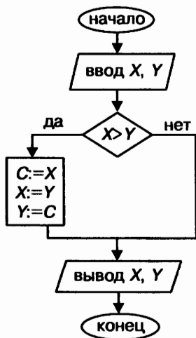
Рис. 6.4. Блок-схема алгоритма упорядочения двух
