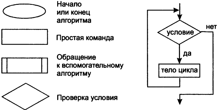
Рис. 5.9. Элементы блок-схем и структура «цикл»
